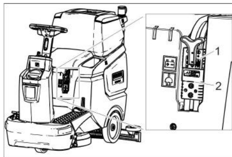
1 电池插头，电池侧
