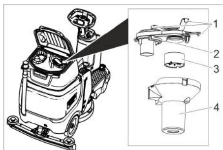
1 Фіксуючі гаки 2 Фільтр для затримування волокон
